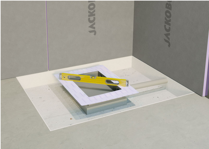
1) Ausrichten und anschließen der Installationsbox
