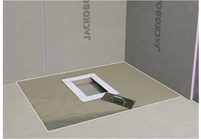
2) Bodenaussparung mit Ausgleichestrich ausfüllen
