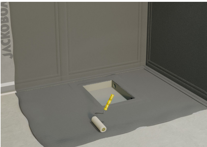
3) Übergänge und Flächen abdichten
