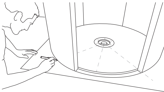
8) Die gewünschte Breite der Eingangsöffnung wird an dem letzten Wandelement angezeichnet ...
